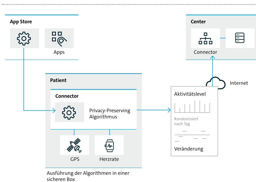
Abbildung 14: Privacy-Preserving Algorithmen: Beispiel
